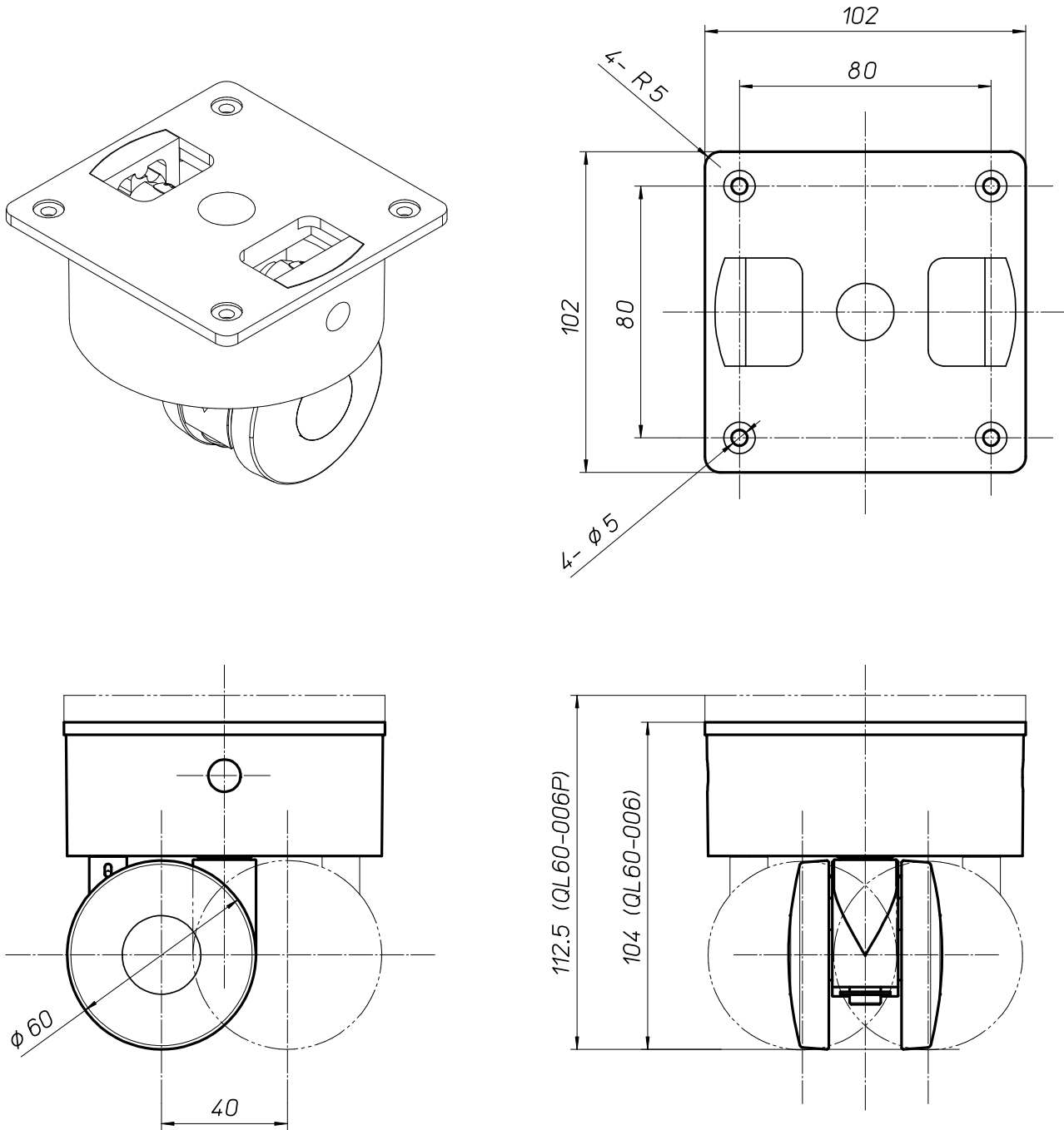
QuadLocks60 補助輪 品番: QL60-006 QL60-006P
